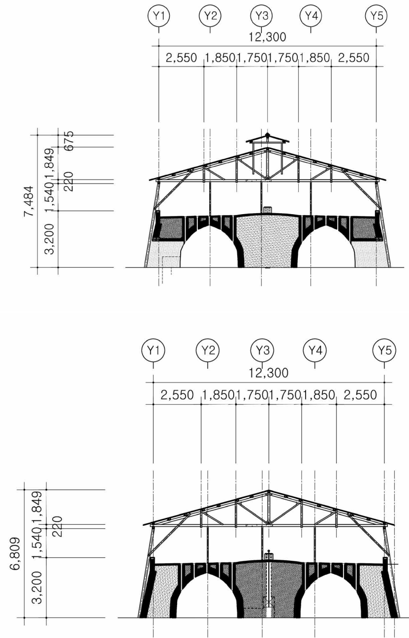
가마 종단면도(수원시, 『수원 영신연와 벽돌공장 일원 기록화사업』, 2020)
