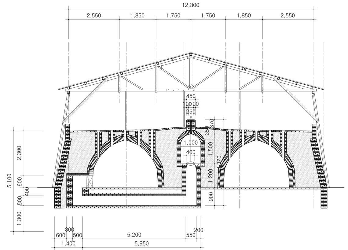
지하로 연결되는 외벽 소연도와 중앙연도(수원시, 『수원 영신연와 벽돌공장 일원 기록화사업』, 2020)
