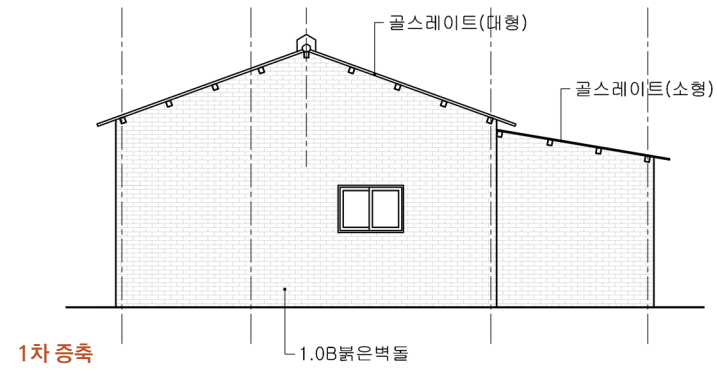
사택 1동 측면도(수원시, 『수원 영신연와 벽돌공장 일원 기록화사업』, 2020)
