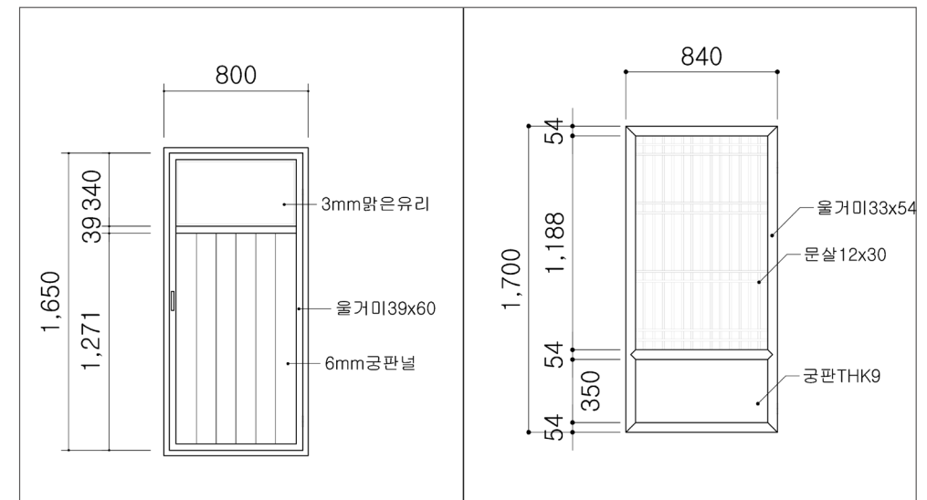
정면 출입문과 거실출입문
