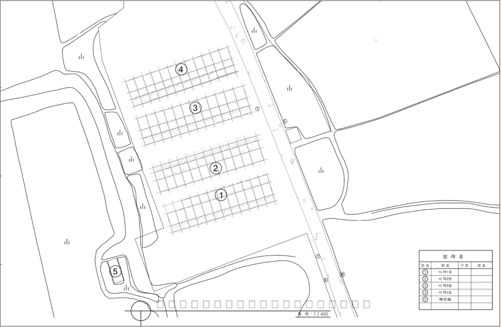
사택 확대 계획배치도(1차 증축, 수원시, 『수원 영신연와 벽돌공장 일원 기록화사업』, 2020)
