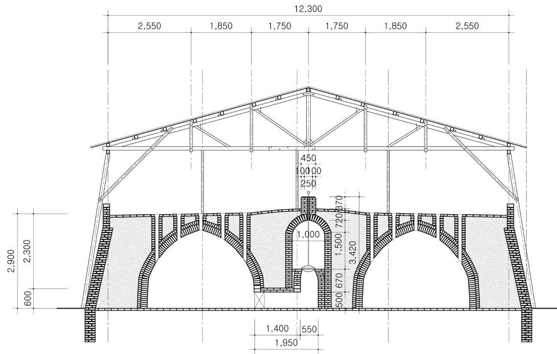
내벽 소연도와 중앙연도 연결(수원시, 『수원 영신연와 벽돌공장 일원 기록화사업』, 2020)
