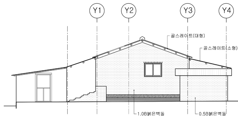
사택 1동 우측면도(현황, 수원시, 『수원 영신연와 벽돌공장 일원 기록화사업』, 2020)
