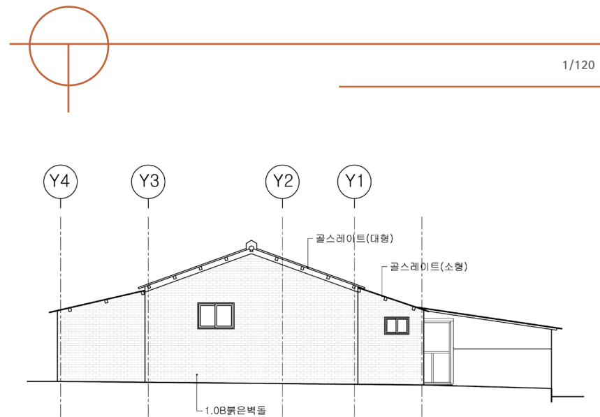
사택 1동 좌측면도(현황)
