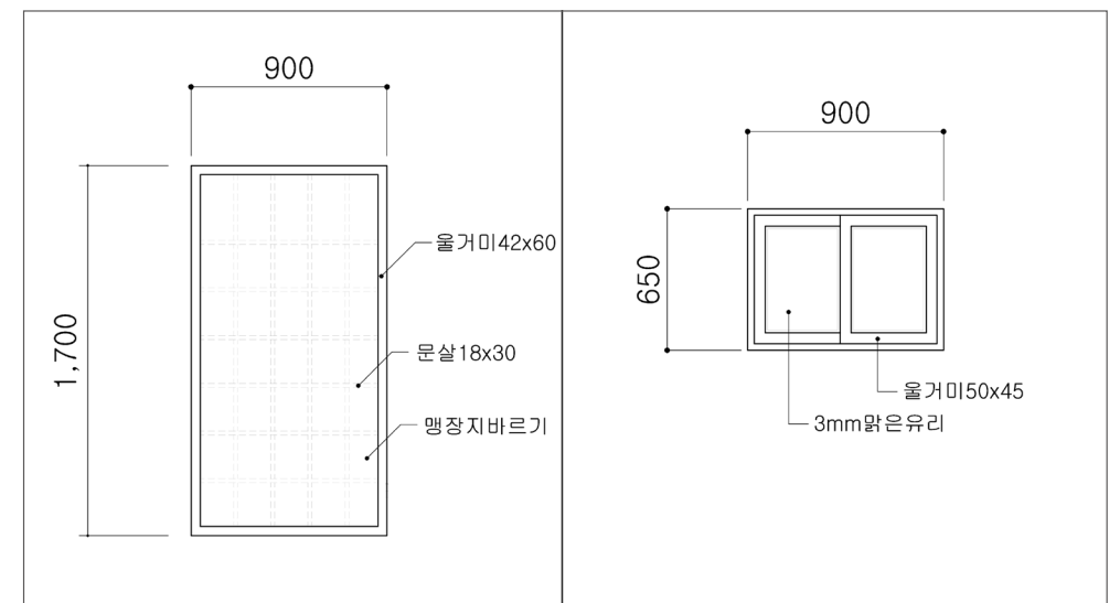
방 출입문과 정면 창(수원시, 『수원 영신연와 벽돌공장 일원 기록화사업』, 2020)
