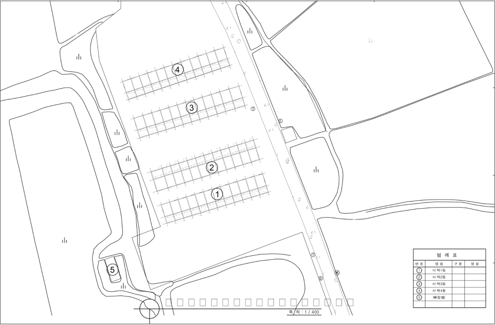
사택 확대 계획배치도(원형, 수원시, 『수원 영신연와 벽돌공장 일원 기록화사업』, 2020)
