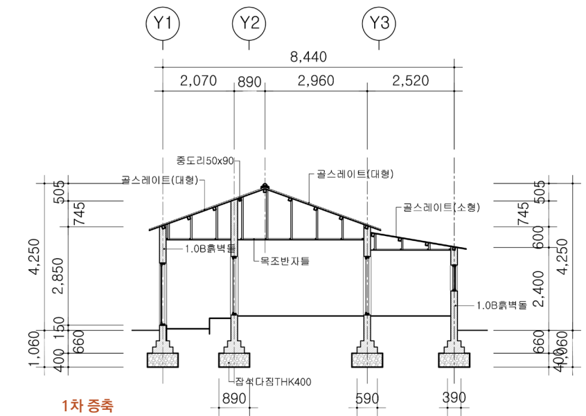
사택 1동 종단면도(수원시, 『수원 영신연와 벽돌공장 일원 기록화사업』, 2020)
