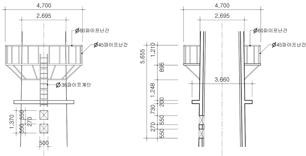
굴뚝 상세도(수원시, 『수원 영신연와 벽돌공장 일원 기록화사업』, 2020)
