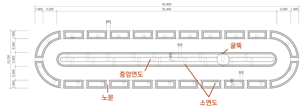
영신연와 가마 하부 평면도(수원시, 『수원 영신연와 벽돌공장 일원 기록화사업』, 2020) 중앙에 대연도가 자리 잡고 있고, 소연도 41좌가 내벽과 외벽에 지그재그식으로 설치되어 있다.
