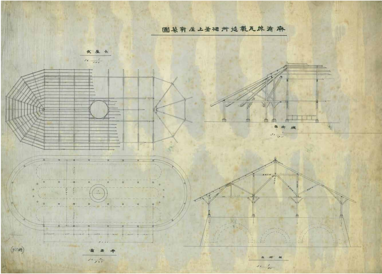
연와제조소 호프만가마 설계도(국가기록원 제공)
