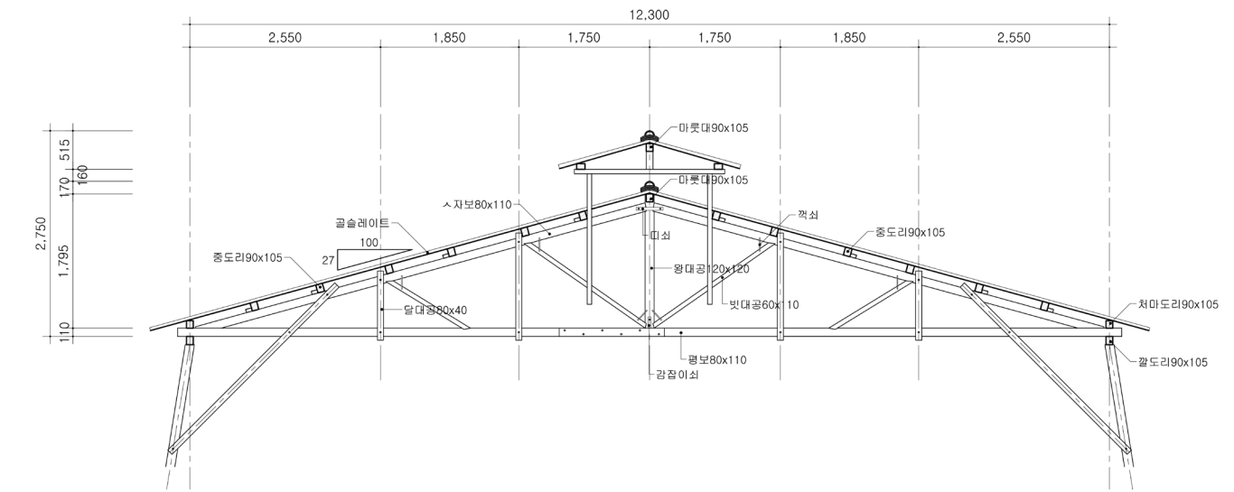
지붕틀 상세도(수원시, 『수원 영신연와 벽돌공장 일원 기록화사업』, 2020)
