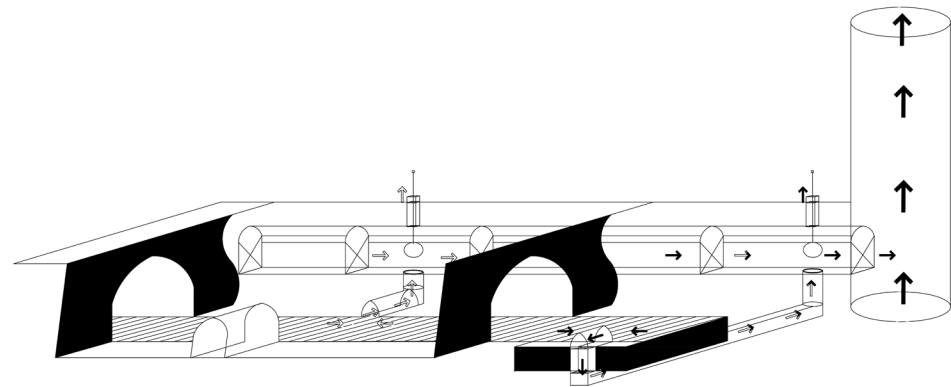
연기의 흐름(수원시, 『수원 영신연와 벽돌공장 일원 기록화사업』, 2020) 댐퍼를 조절하면 내벽과 외벽에 설치된 소연도를 통해 연기가 모여져 중앙연도를 거쳐 굴뚝으로 빠져나간다.
