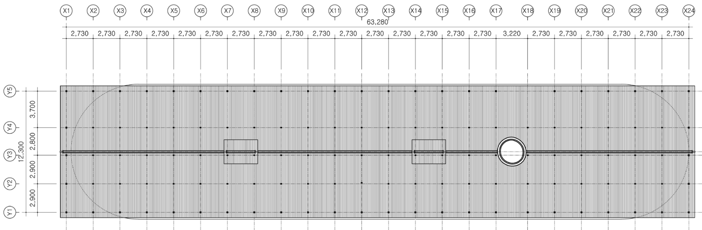
지붕 평면도(수원시, 『수원 영신연와 벽돌공장 일원 기록화사업』, 2020)
