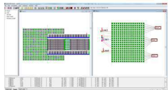
그림 2-14 | buildingEXODUS 구동화면
