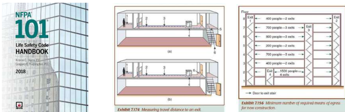
그림 2-7 | NFPA101 매뉴얼
