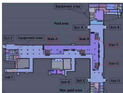
그림 2-23 | 역 홀 개략도
