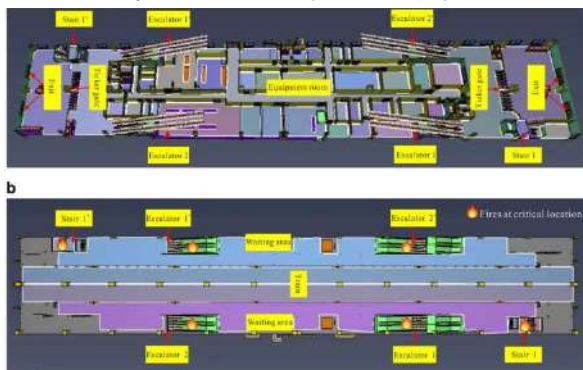
그림 2-21 | 플랫폼 및 역 홀의 개략도
