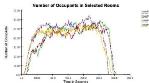
그림 2-28 | 각 계단의 흐름-시간 차트
