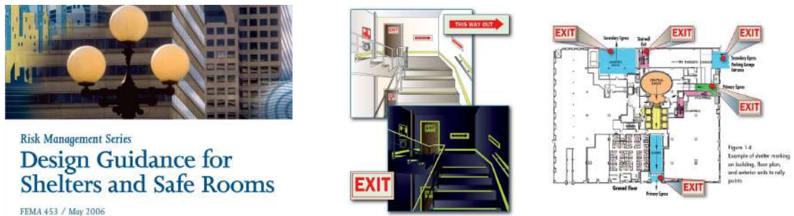
그림 2-4 | FEMA453 매뉴얼
