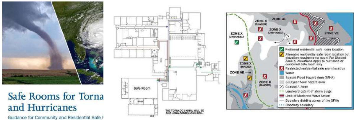
그림 2-1 | FEMA361 매뉴얼
